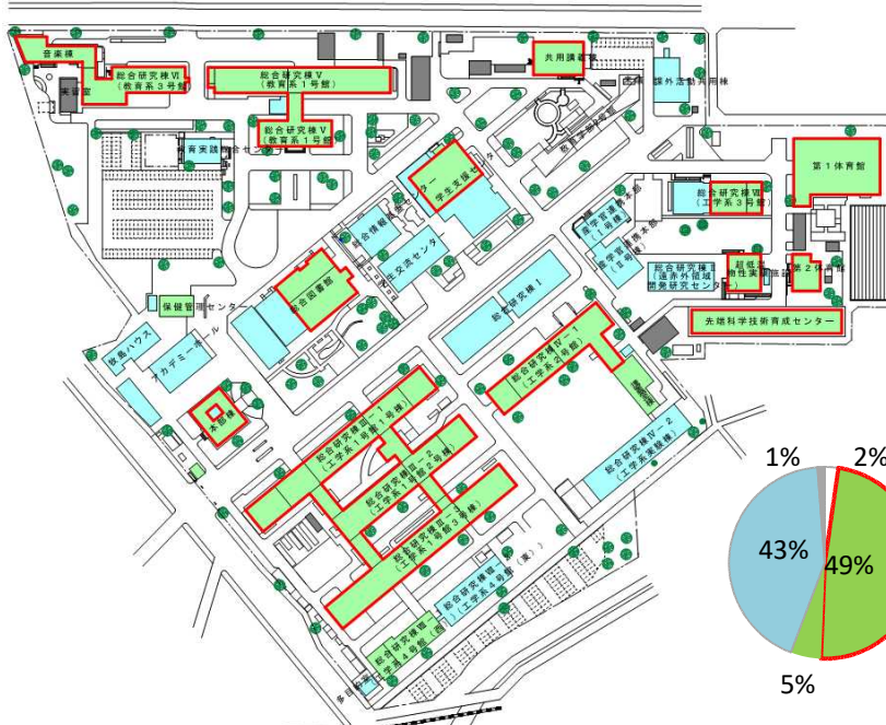
【各建物の耐震性能】
