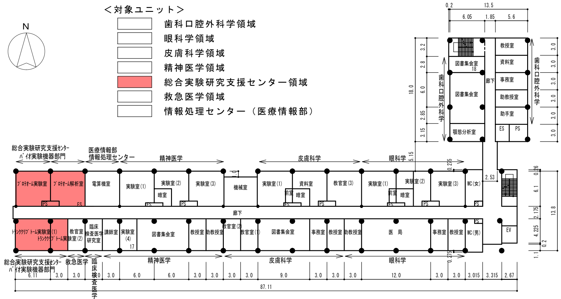
(臨床研究棟) 2階平面図 1:400
