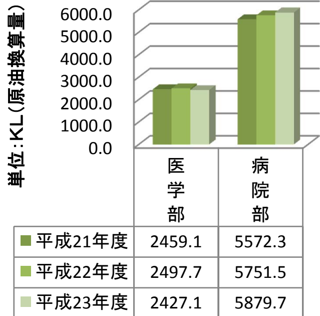
総エネルギー(電気+熱量)使用量 月累計(04月~03月)
